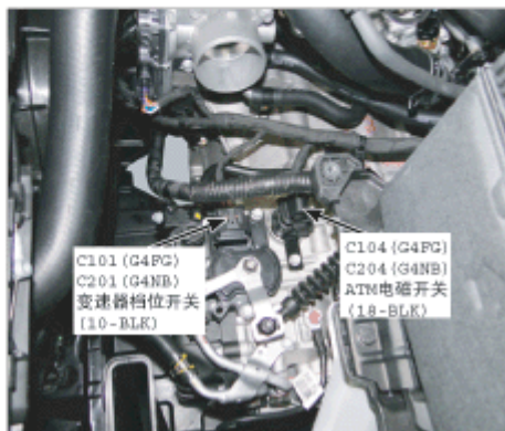
39. 变速器顶部
