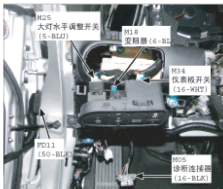
40. 仪表板左侧
